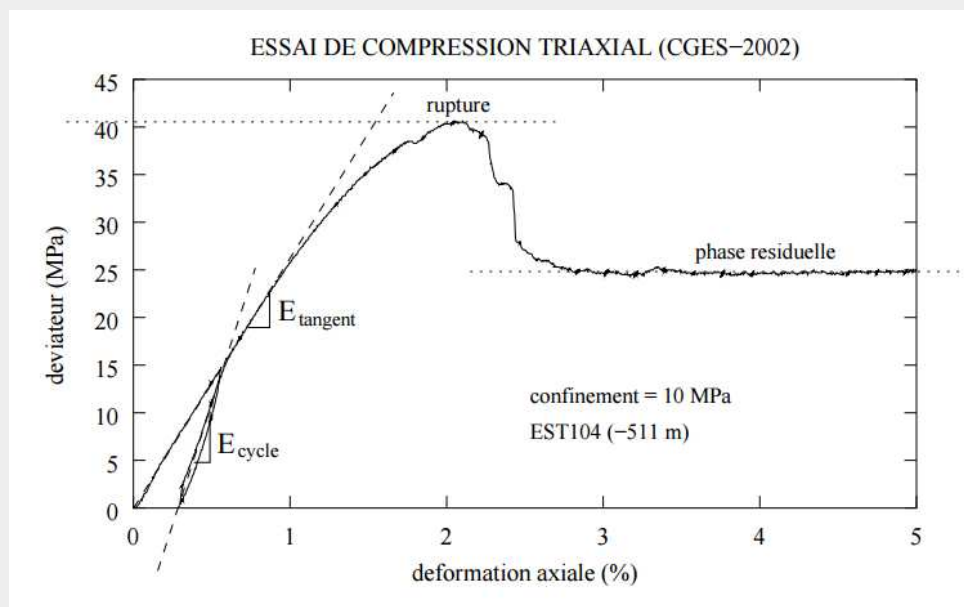
Figure 2.5: Deviator stress (deviateur) against axial deformation (déformation axiale) (Miehe, 2004).
